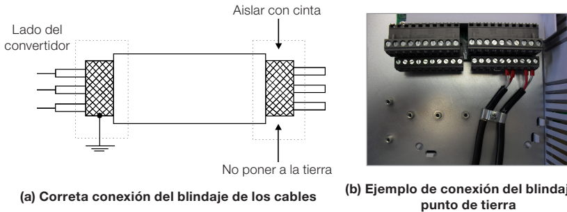
Figura 3.7: (a) y (b) Conexión del blindaje
