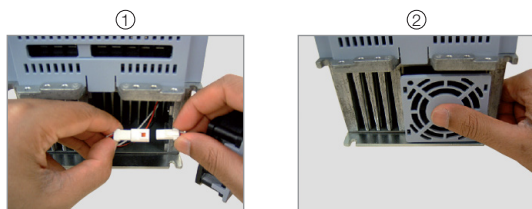
Figura 6.1: (a) y (b) Retirada del ventilador del disipador
