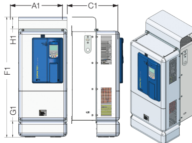
Frame size E 180 and 211 A with Nema1 kit Tamaño E 180 y 211 A con kit Nema1 Mecânica E 180 e 211 A con kit Nema1
